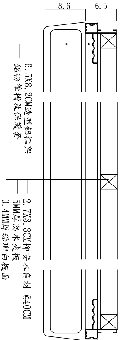
平面圖 S:1/5
